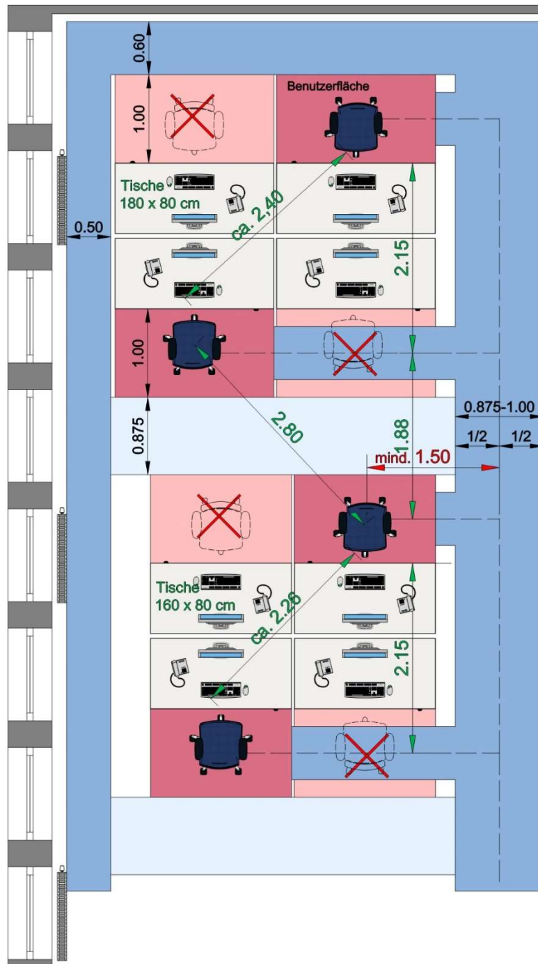
Abbildung 3: Bildschirmarbeitsplätze in 4er-Blockanordnung ohne Änderung des bestehenden Verkehrsweges von 0,875 m zwischen den Blöcken
